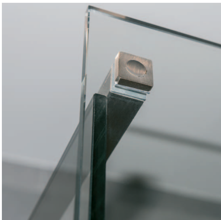
Raidisseur carré Mur-Glace et Glace-Glace – Inox brossé 20x20.
